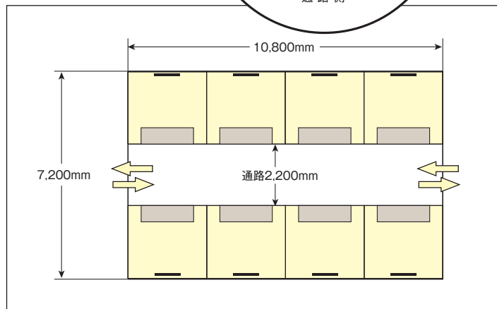
小間配置図(テント1張あたり)
