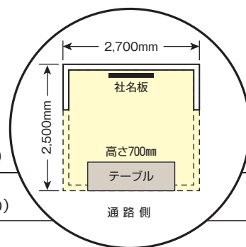
基礎小間 平面図(予定)
